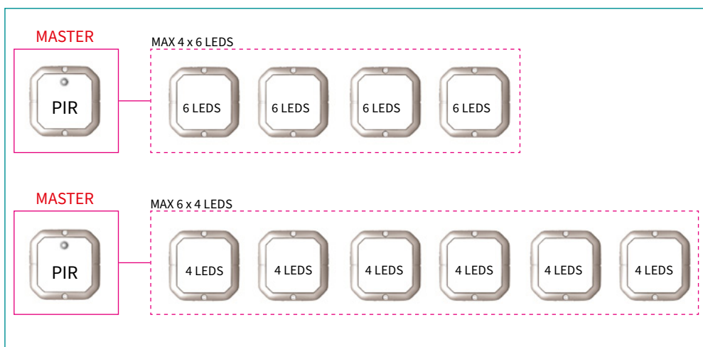
Exemple de montage Maître (PIR) + Esclaves - Assembly suggestion Master (PIR) + Slaves - Montagebeispiel Meister (PIR) + Sklave
